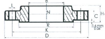
ISO PN 20 - Série 150 lbs - ASME B 16.5
